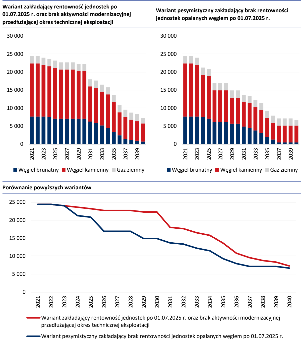
Rys. 3-9 Osiągalna moc netto w istniejących jednostkach konwencjonalnych biorących udział w mechanizmie centralnego bilansowania [MW]
