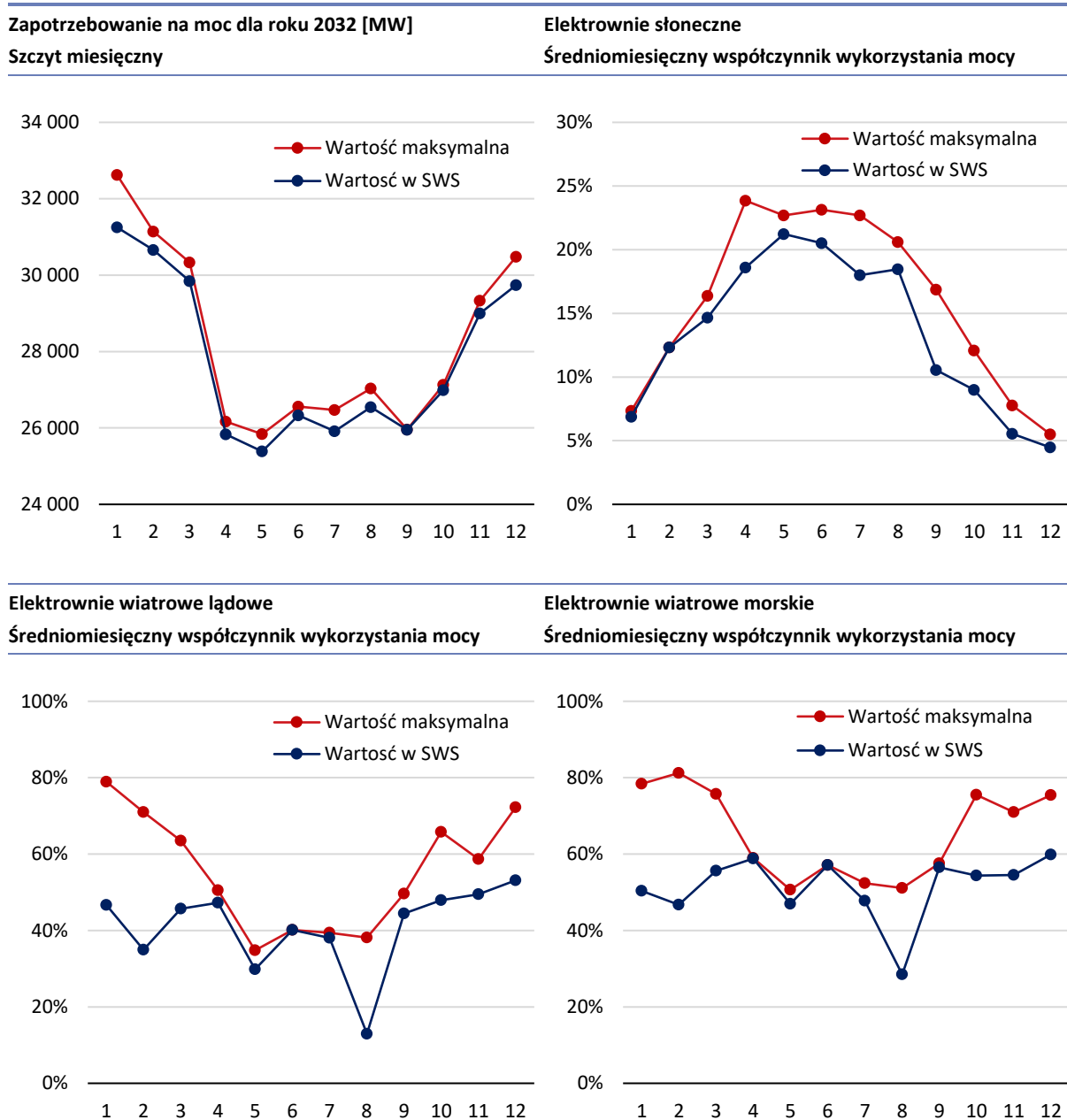
Rys. 4-2 Porównanie maksymalnych wartości zapotrzebowania oraz współczynnika wykorzystania mocy OZE z wartościami roku klimatycznego SWS
