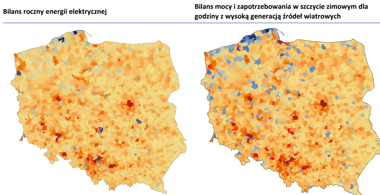
Rys. 4-10 Rozkład przestrzenny generacji i zapotrzebowania w podziale na gminy – 2032 r.
