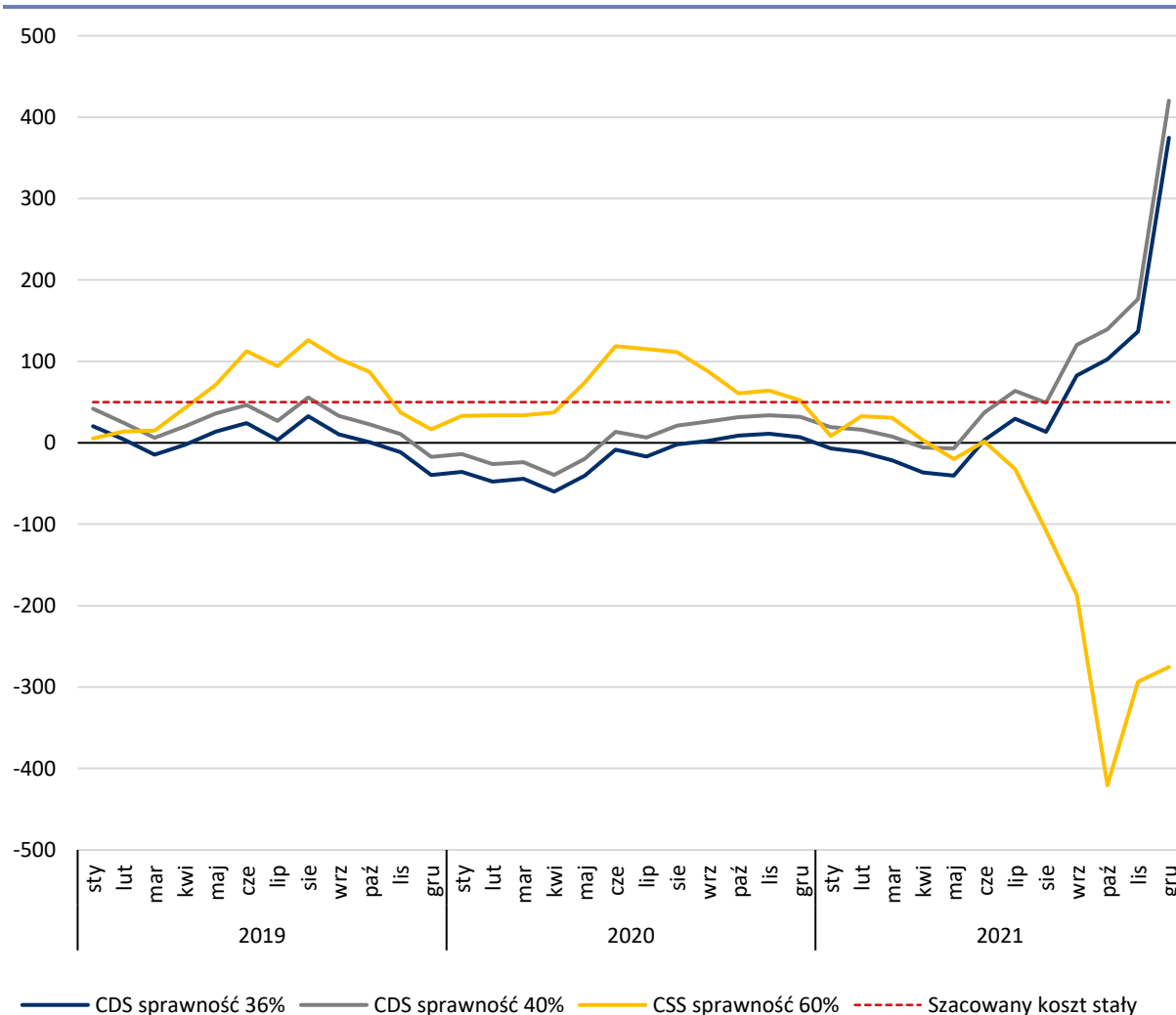
Rys. 3-16 CSS i CDS dla poszczególnych typów źródeł wytwórczych [PLN/MWh]
