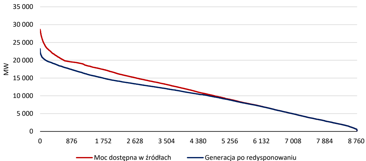
Rys. 4-11 Rzeczywista moc generacji ze źródeł fotowoltaicznych, lądowych i morskich elektrowni wiatrowych oraz moc dostępna, wynikająca z energii pierwotnej, w wariantach bazowym, w roku 2032 i roku klimatycznym SWS
