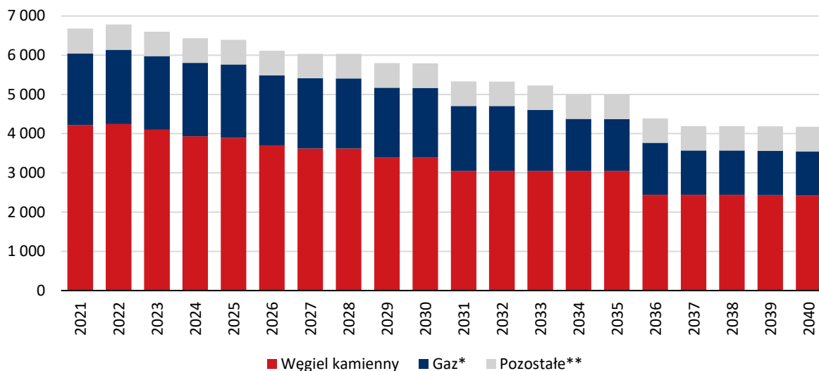
Rys. 3-10 Osiągalna moc netto w istniejących jednostkach konwencjonalnych niebiorących udziału w centralnym bilansowaniu. Stan na koniec roku [MW]
